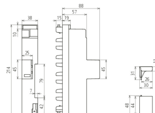
Maßbild DSH ZP 2 TT 255
