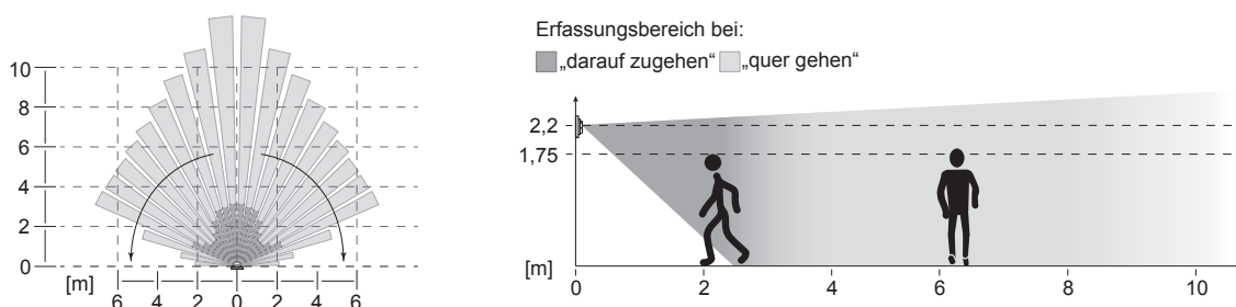
Bild 7: Erfassungsbereich des Bewegungsmelders bei Montagehöhe 2.2 m
