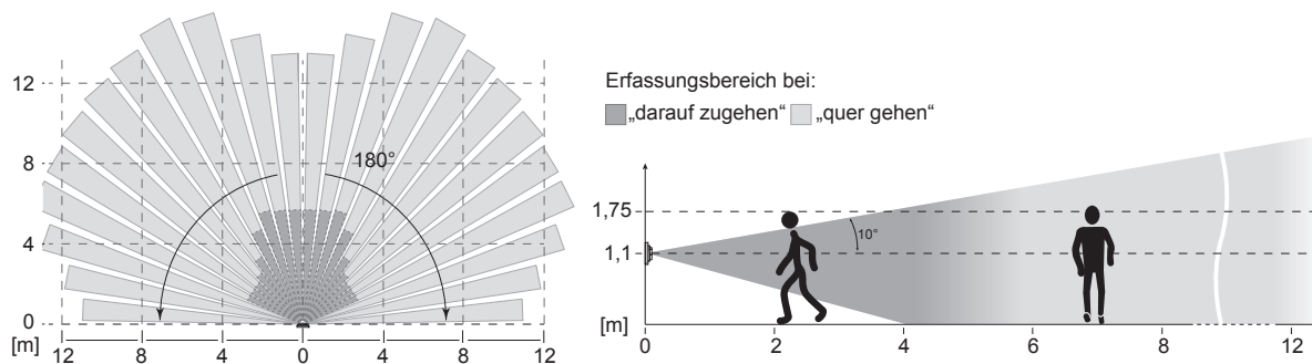
Bild 6: Erfassungsbereich des Bewegungsmelders bei Montagehöhe 1.1m
